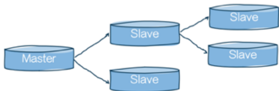
主从复制
